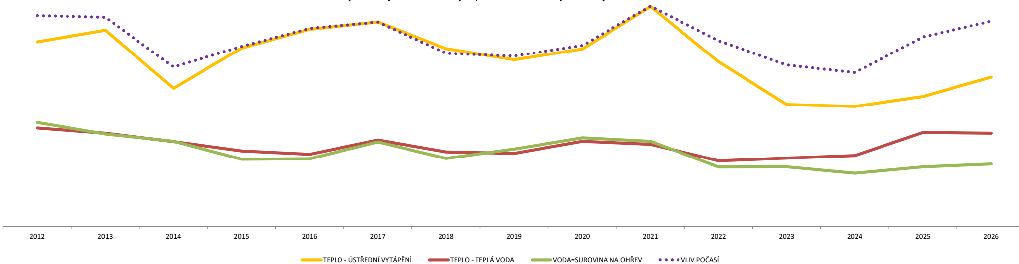
Sledování spotřeby TEPLA na vytápění a ohřev teplé vody v letech ZA CELÝ DŮM
